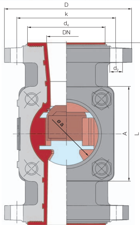
Baureihe SRZ-V mit Rückschlag-Hohlkegel und weichdichtendem Sitz aus Fluorkautschuk (z. B. Kalrez®)
